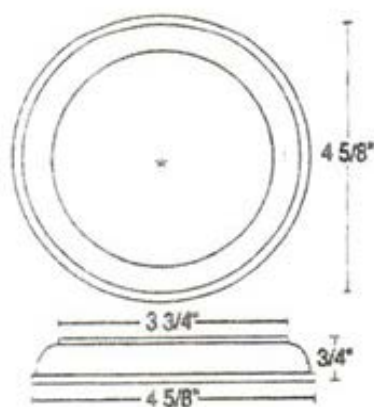
7317 Round Rosette
